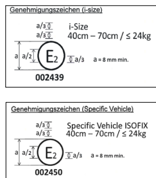
Abbildung 3 Genehmigungszeichen ECE-Reglement Nr. 129
